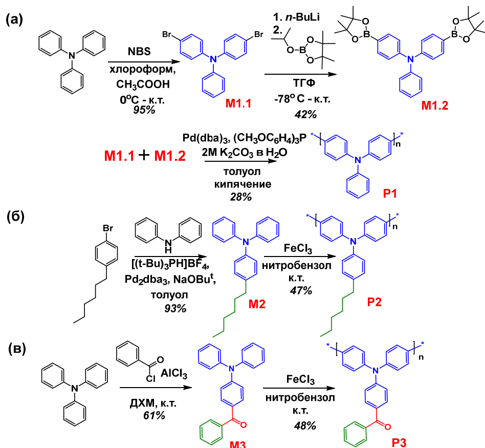
Рисунок 3.1.4 – Схема синтеза модельных полимеров на основе ТФА P1 (а), P2 (б), P3 (в)
