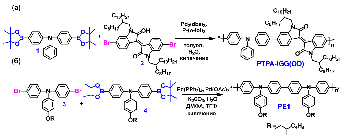
Рисунок 1.3.2 – Схема синтеза полимеров на основе ТФА методом поликонденсации по Сузуки
