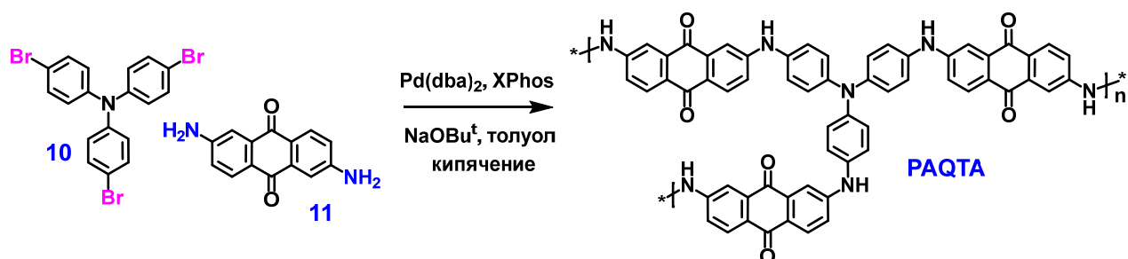
Рисунок 1.3.6 – Схема синтеза полимеров на основе ТФА методом поликонденсации по Бухвальду-Хартвигу
