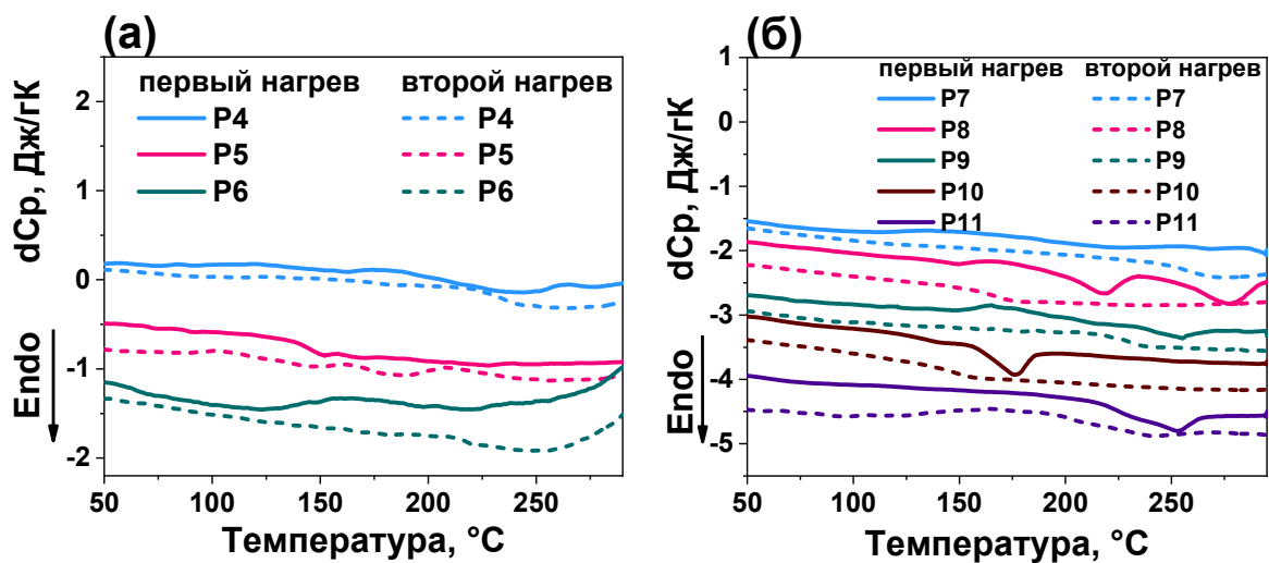
Рисунок 4 – Кривые ДСК первого и второго нагрева полимеров P4–P6 (а) и полимеров P7–P11 (б)
