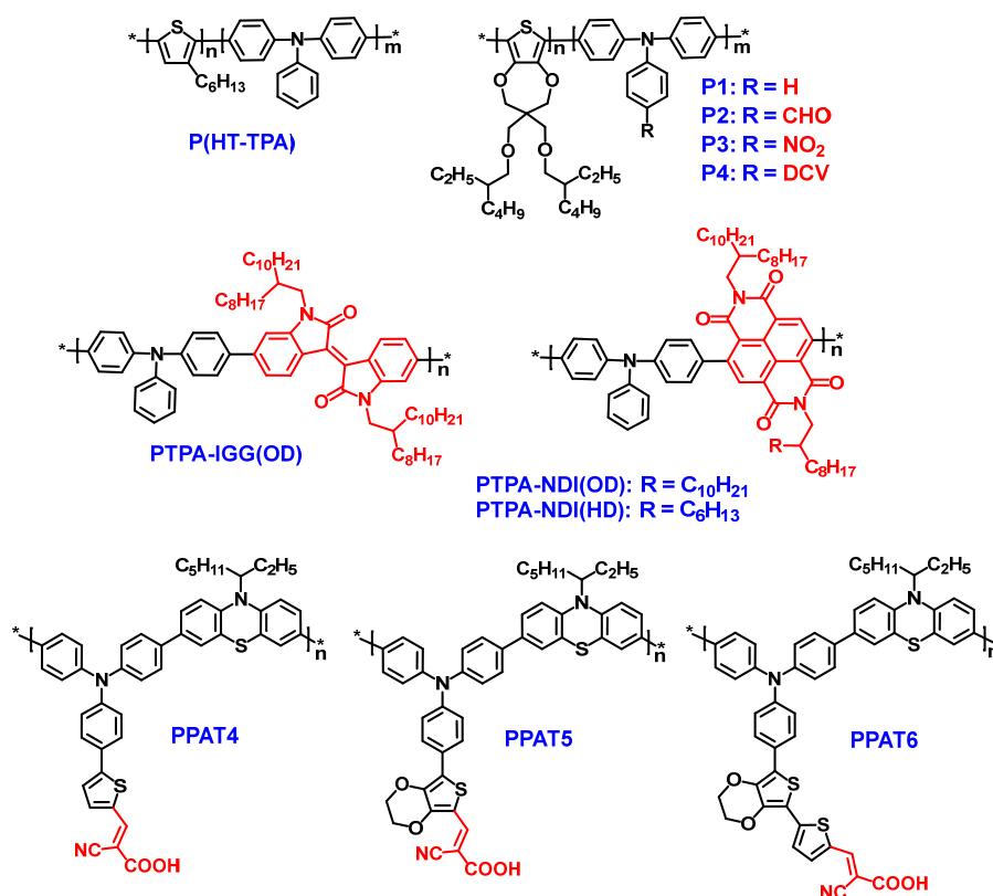
Рисунок 1.2.3 – Структурные формулы сополимеров на основе ТФА
