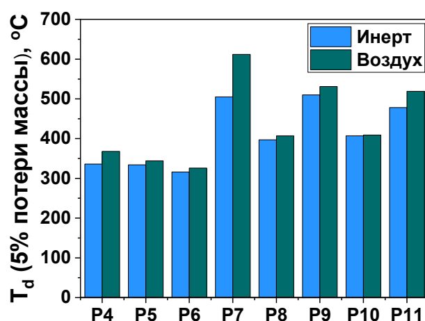
Рисунок 3.2.5 – Диаграмма температур деструкции полимеров с цианоэфирными и дициановинильными ЭА группами в инертной атмосфере и на воздухе
