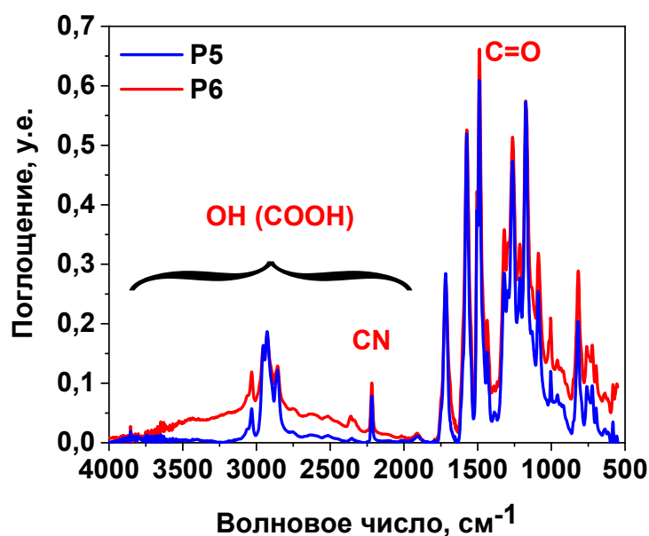
Рисунок 3.1.7 – ИК-Фурье спектр полимеров P5 и P6
