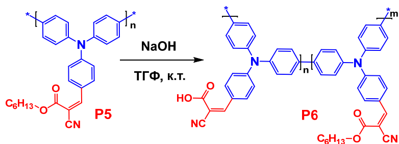
Рисунок 3.1.6 – Схема синтеза сополимера с цианокрбоксильной ЭА группой
