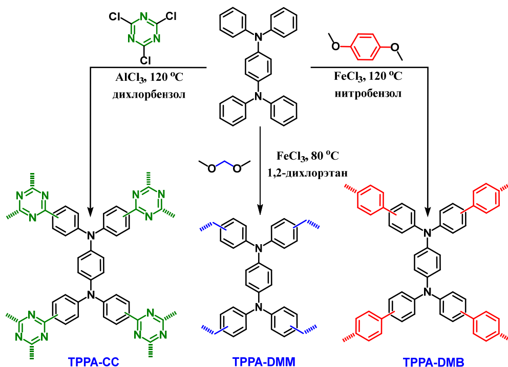
Рисунок 1.3.13 – Схема синтеза полимеров на основе ТФА методом ацилирования по Фриделю-Крафтсу
