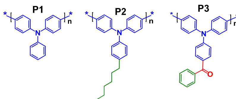
Рисунок 3.2.1 – Структуры модельных полимеров на основе ТФА
